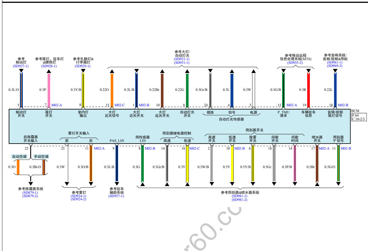
车身控制模块(BCM)系统(2)
